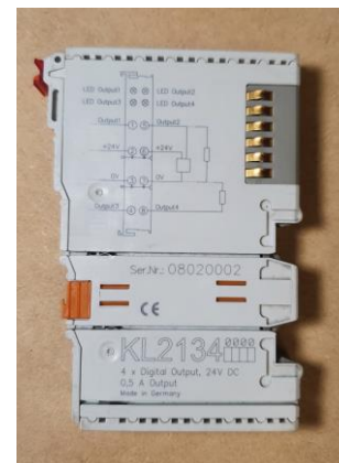
BECKHOFF KL2134
