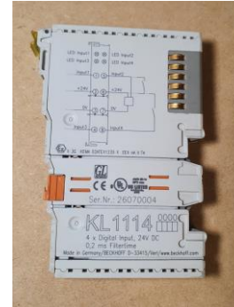
BECKHOFF KL1114
